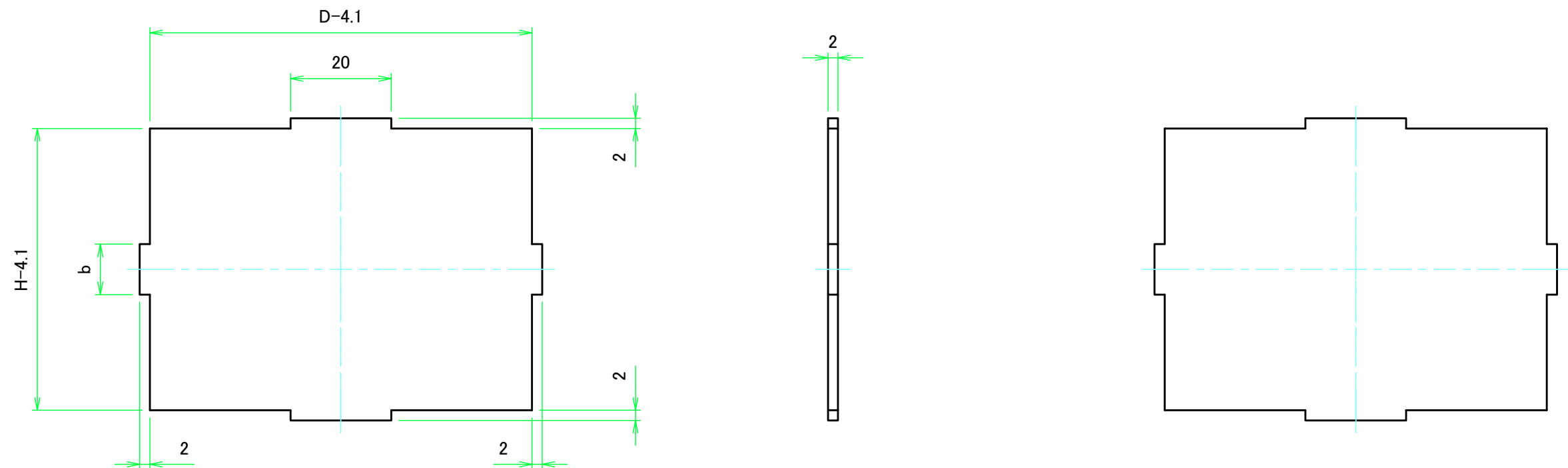
Dパネル1表面 / D panel 1 Frontside
